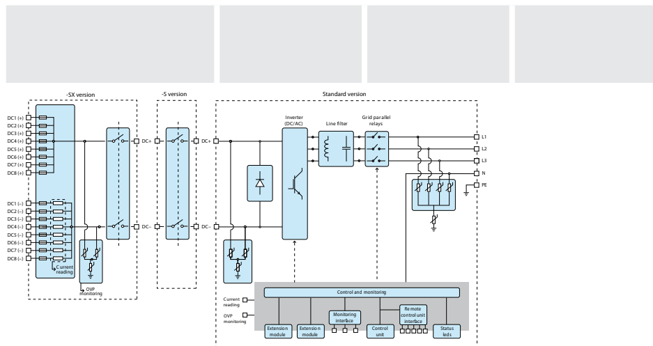
Блок-диаграмма PRO-33.0-TL-OUTD
