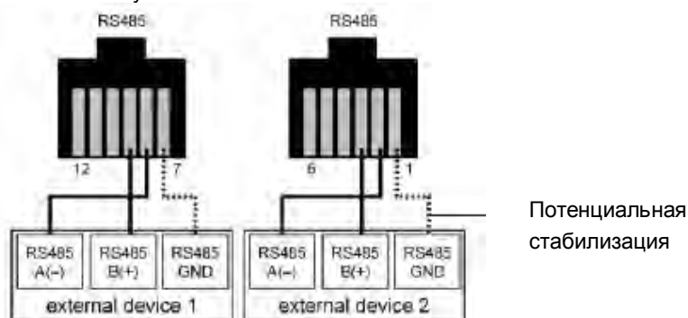
Рисунок 29: RS485 интерфейс модуля VARIOMOD XC
