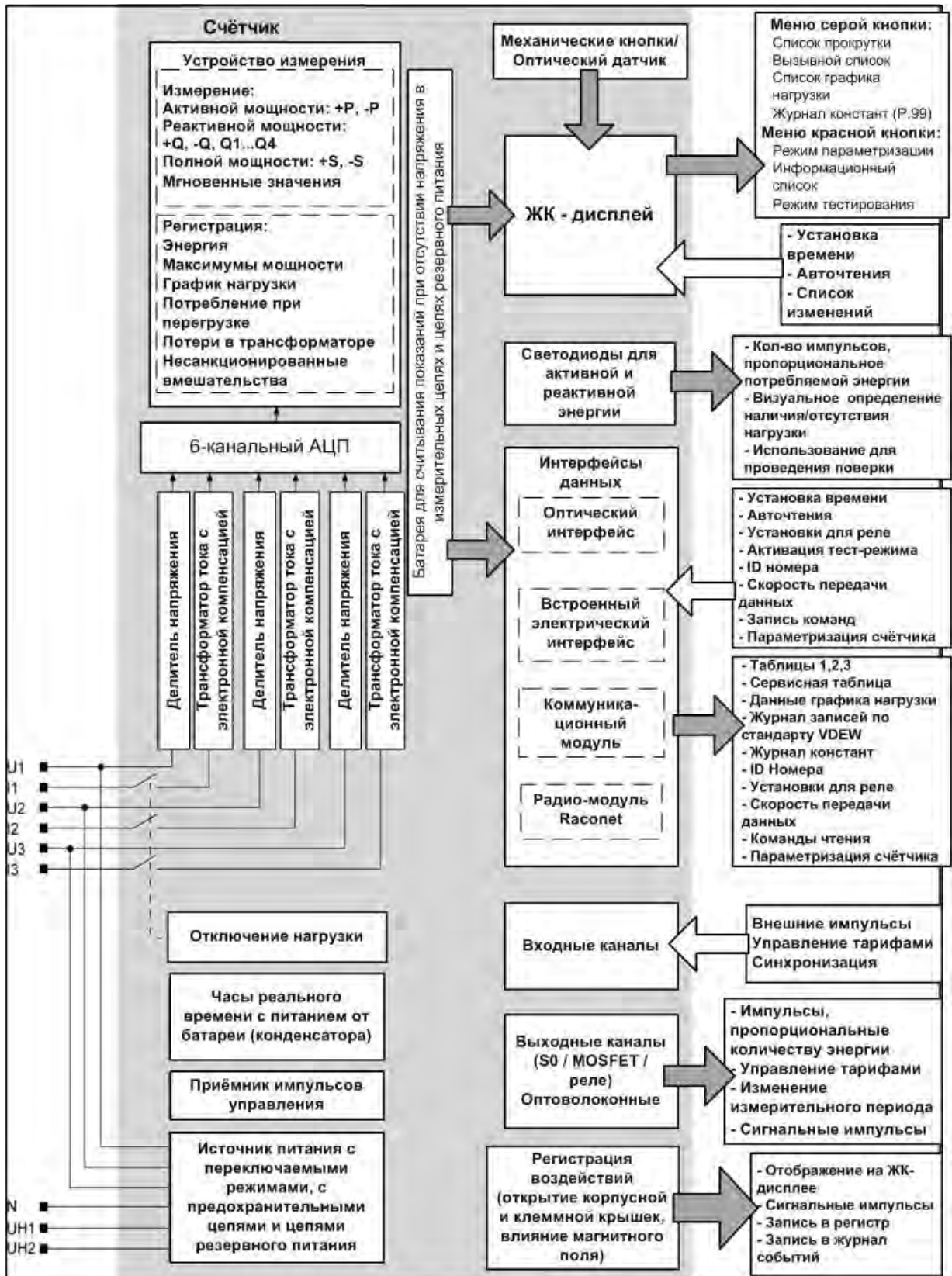
Рисунок 12: Блок-схема счетчика
