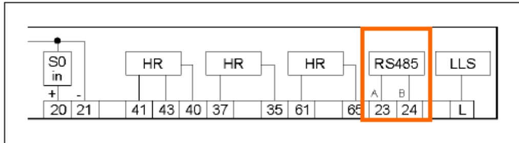
Рисунок 19: Диаграмма связей - RS485
