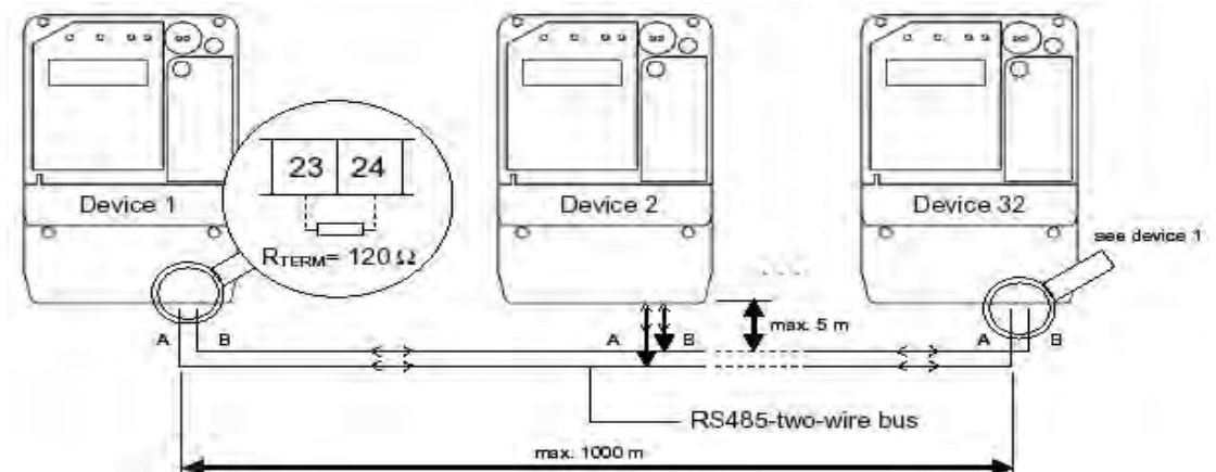
Рисунок 21: RS-485-двухпроводная система шины
