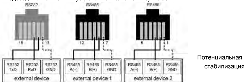
Рисунок 30: Интерфейсы Модуля интерфейса XC
