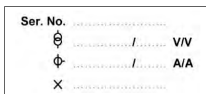
Рисунок 15: Маркировка трансформатора
