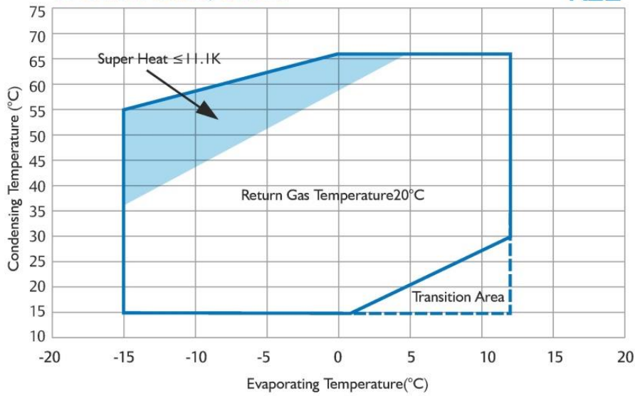
YM34A-YM210A, 2-13HP
