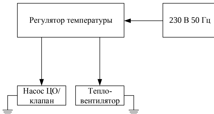
Рисунок 1 – Схема подключения AIR LOGIC FAN
