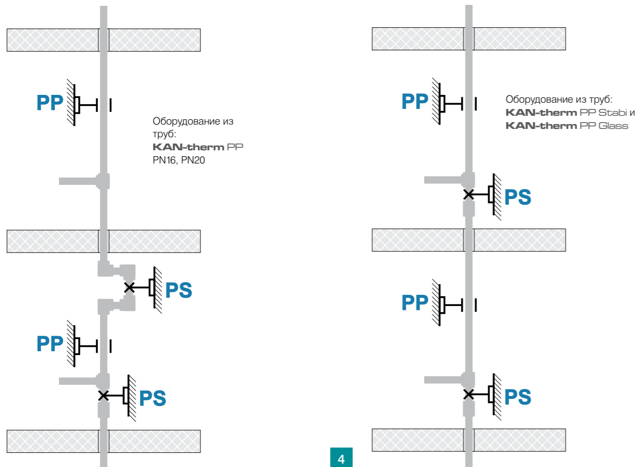
Примеры прокладки стояков горячего водоснабжения в зависимости от вида труб (рис. 3 и 4), где: PP - подвижная опора, PS - точка неподвижной опоры
