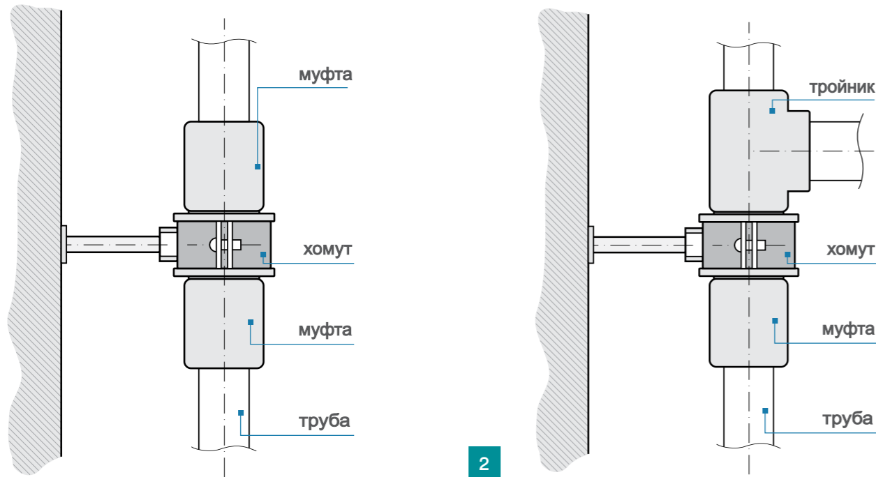
Точки неподвижной опоры - примеры (рис. 1 и 2)
