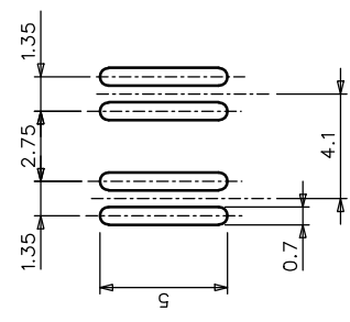
Particolare E scala 5/1 Sez.bruciatore:237.65mm 2
