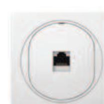
E616S.00 Priključnica komunikacijska sa Keystone modulom RJ45 Cat6A FTP Data socket with Keystone module RJ45 Cat6A FTP
