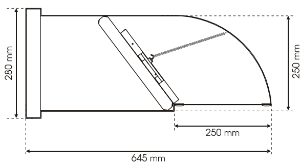
i Размеры приточного устройства MAXI
