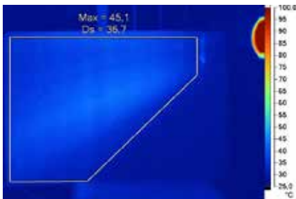
Wärmebild bei 50 cm Abstand. Maximaltemperatur: 45,1° C
