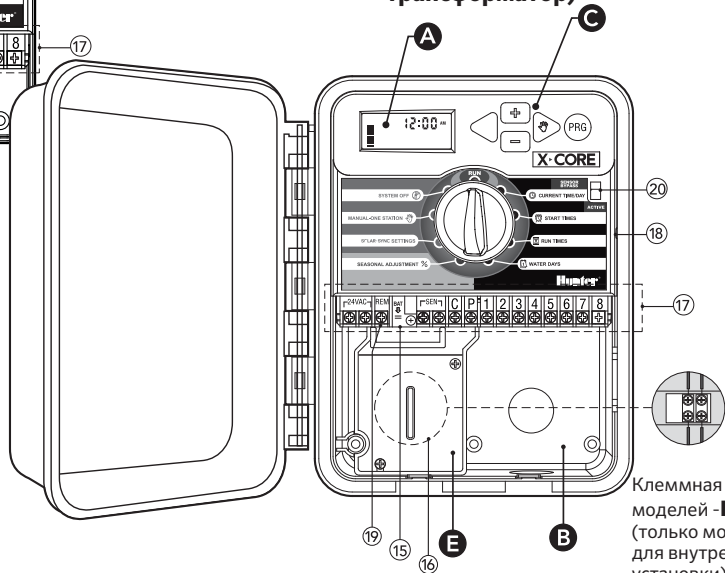
Модель для наружной установки (включая встроенный трансформатор)
