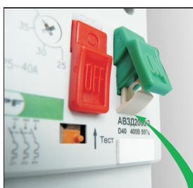
запобіжник від випадкового включення
