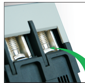
клеми підключення з напайкою контактів
