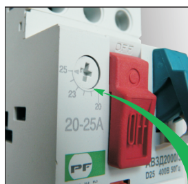
регулятор теплового захисту
