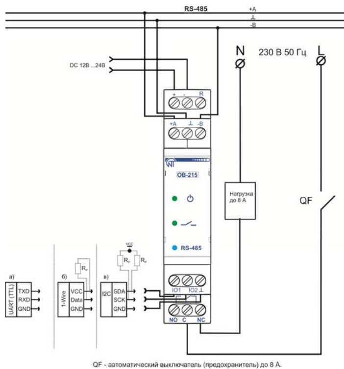
Рисунок 3 – Схема подключения в режиме преобразования интерфейсов
