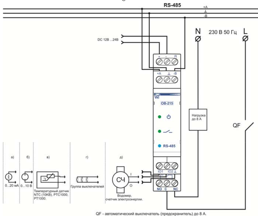
Рисунок 2 – Схема подключения в режиме измерений
