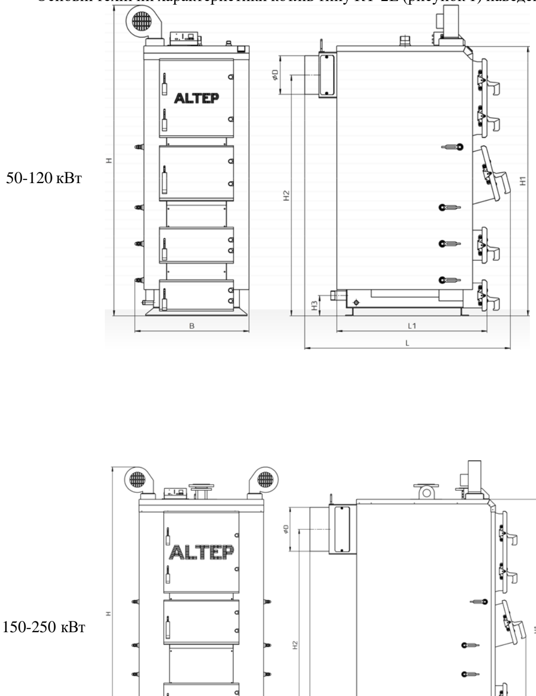
Рисунок 1 – Габаритне креслення котла типу КТ-2Е
