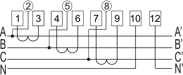
Додаток Д Схема підключення лічильника до мережі живлення в експлуатації
