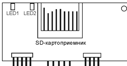
Рисунок 4. Расположение светодиодов на плате «VID-Universal»
