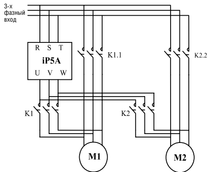
[Схема выключения для режима 2]
