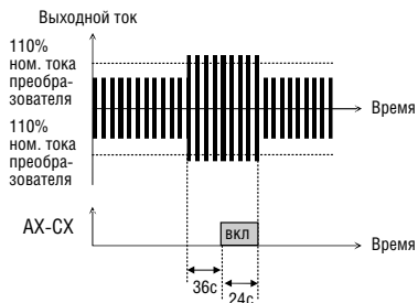
[АХ-СХ, установка 'IOL']
