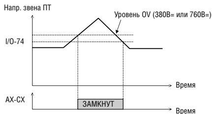
[АХ-СХ, установка 'OV']
