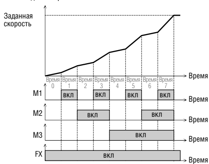
[Работа с различным временем разгона]
