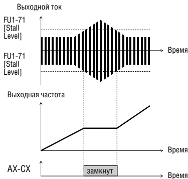
[АХ-СХ, установка 'Stall']
