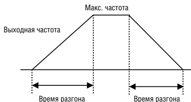
[FU1-73: Макс. частота]
