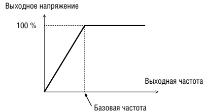
[V/F Характеристика: 'Linear']
