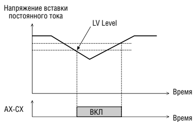
[АХ-СХ, установка 'LV']
