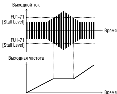
[Токоограничение при разгоне]
