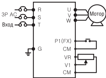
Схема подключения
