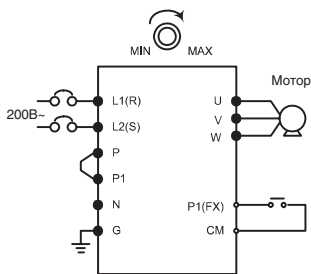
Схема подключения
