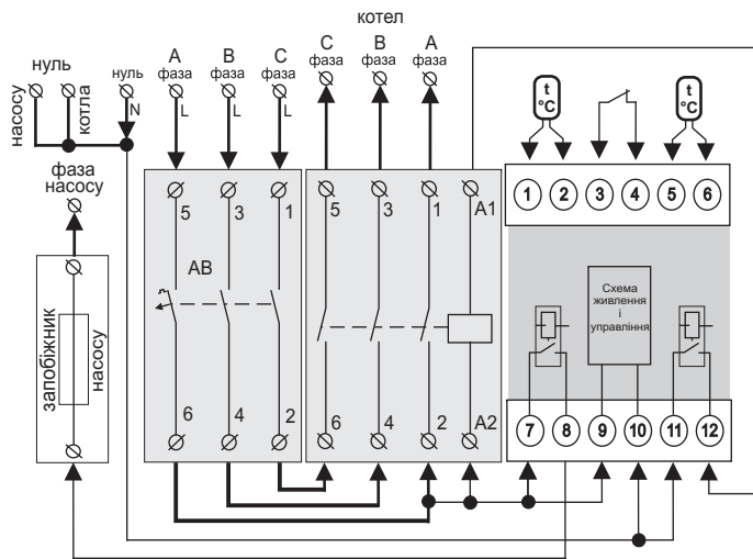
Схема 3. Схема підключення автоматики 3-фазного котла.
