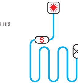
Схема укладки двожильного кабелю TXLP/2R
