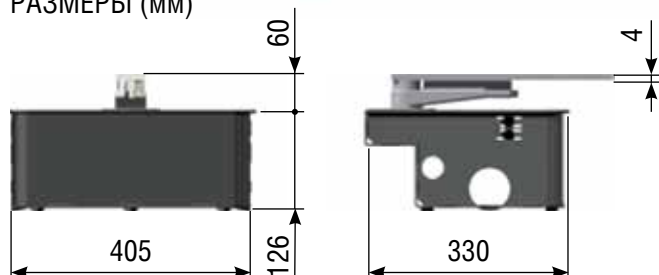
РАЗМЕРЫ (мм)
