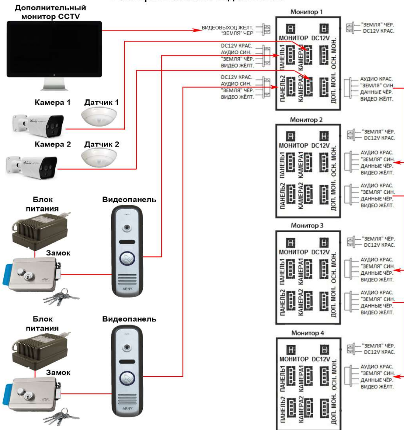
Расширенная схема подключения
