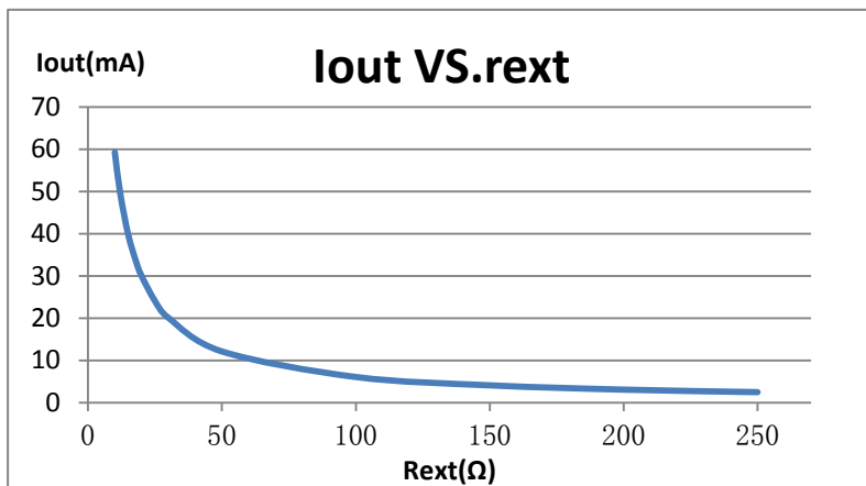
图 1. SM2082D 输出电流与 Rext 电阻关系曲线
