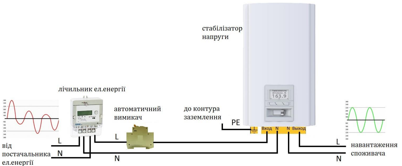
Рисунок 7. Схема підключення стабілізатора до однофазної мережі
