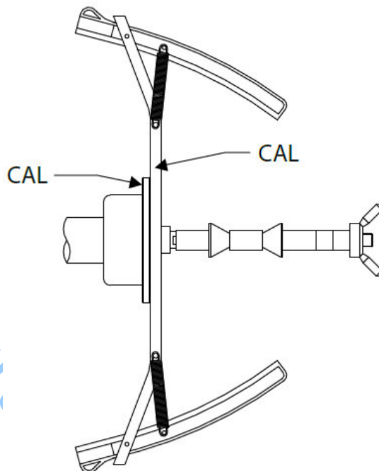
Рис. 4.1 - Применение фланца для мотоколес на вал. Совместите надписи "CAL" на фланце станда и на фланце для мотоколес
