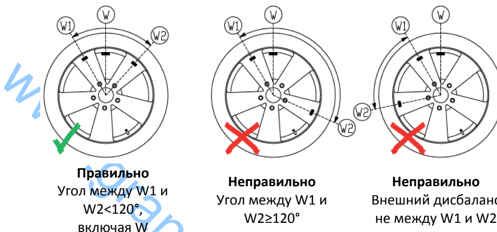
Рис.6.1 – Правильное и неправильное расположение скрытых грузиков
