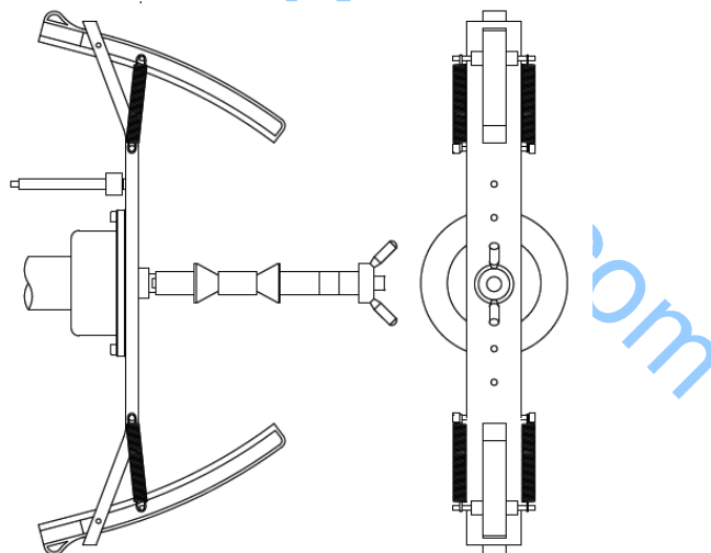
Рис. 4.3 - Применение образцового грузика на внешней стороне фланца для мотоколес на валу (фаза Cal3)
