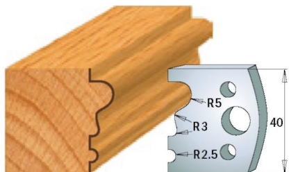
Пара ножів 690.033 Пара обмежувачів 691.033
