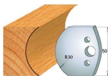
Пара ножів 690.544 Пара обмежувачів 691.544
