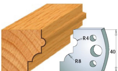
Пара ножів 690.024 Пара обмежувачів 691.024
