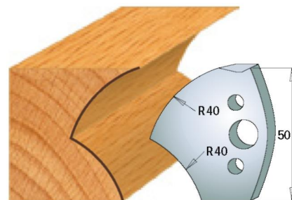
Пара ножів 690.550 Пара обмежувачів 691.550
