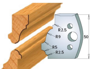
Пара ножів 690.558 Пара обмежувачів 691.558
