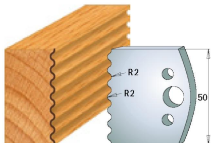
Пара ножів 690.552 Пара обмежувачів 691.552
