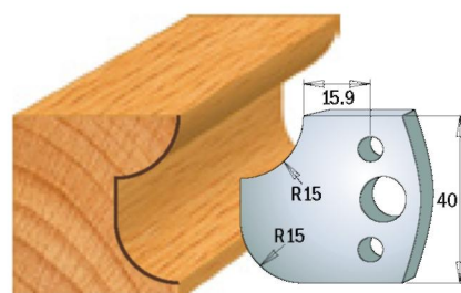
Пара ножів 690.177 Пара обмежувачів 691.177
