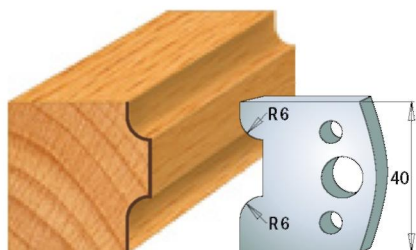
Пара ножів 690.063 Пара обмежувачів 691.063
