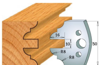
Пара ножів 690.523 Пара обмежувачів 691.523
