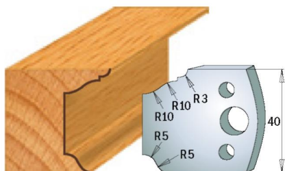
Пара ножів 690.079 Пара обмежувачів 691.079
