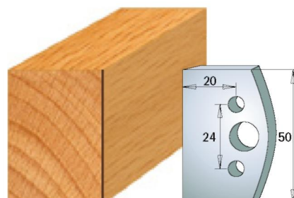
Пара ножів 690.500 Пара обмежувачів 691.500
