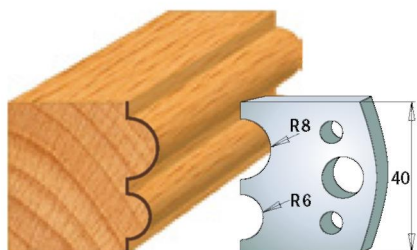
Пара ножів 690.051 Пара обмежувачів 691.051
