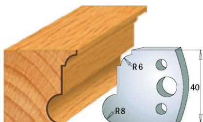
Пара ножів 690.054 Пара обмежувачів 691.054
