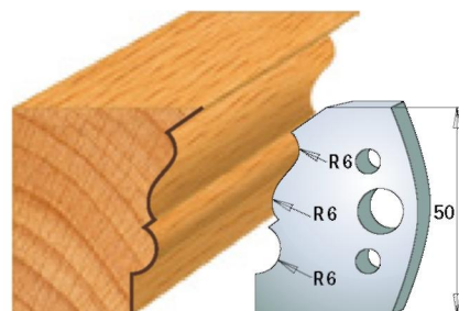
Пара ножів 690.509 Пара обмежувачів 691.509
