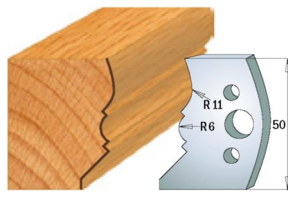
Пара ножів 690.503 Пара обмежувачів 691.503
