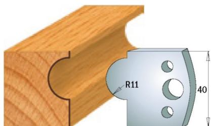
Пара ножів 690.093 Пара обмежувачів 691.093
