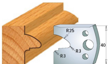
Пара ножів 690.078 Пара обмежувачів 691.078
