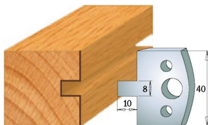
Пара ножів 690.094 Пара обмежувачів 691.094
