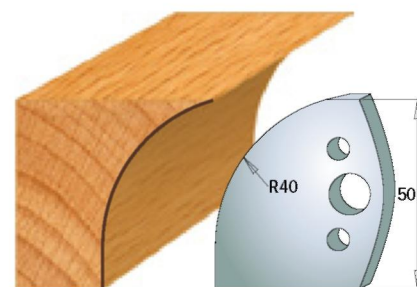
Пара ножів 690.565 Пара обмежувачів 691.565
