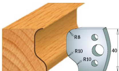
Пара ножів 690.049 Пара обмежувачів 691.049
