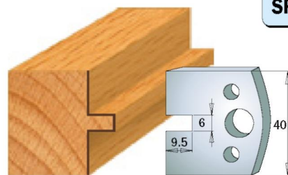
Пара ножів 690.017 Пара обмежувачів 691.017
