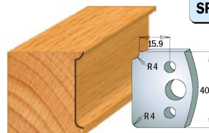
Пара ножів 690.171 Пара обмежувачів 691.171
