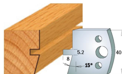
Пара ножів 690.086 Пара обмежувачів 691.086
