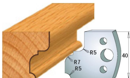
Пара ножів 690.082 Пара обмежувачів 691.082
