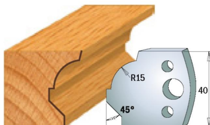
Пара ножів 690.037 Пара обмежувачів 691.037
