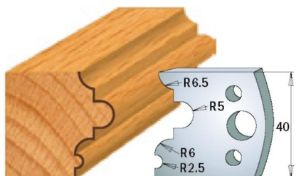
Пара ножів 690.036 Пара обмежувачів 691.036
