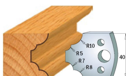
Пара ножів 690.022 Пара обмежувачів 691.022
