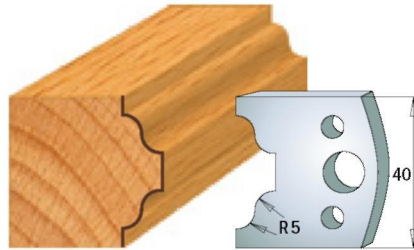
Пара ножів 690.025 Пара обмежувачів 691.025
