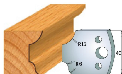
Пара ножів 690.044 Пара обмежувачів 691.044
