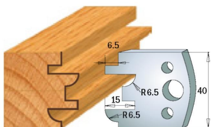
Пара ножів 690.096 Пара обмежувачів 691.096
