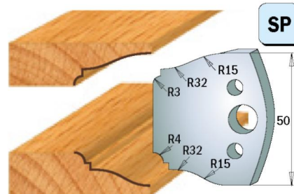
Пара ножів 690.568 Пара обмежувачів 691.568
