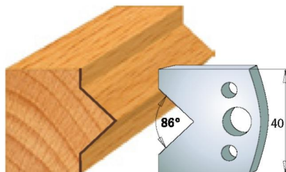
Пара ножів 690.034 Пара обмежувачів 691.034
