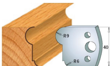
Пара ножів 690.055 Пара обмежувачів 691.055
