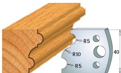
Пара ножів 690.052 Пара обмежувачів 691.052
