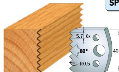
Пара ножів 690.077 Пара обмежувачів 691.077
