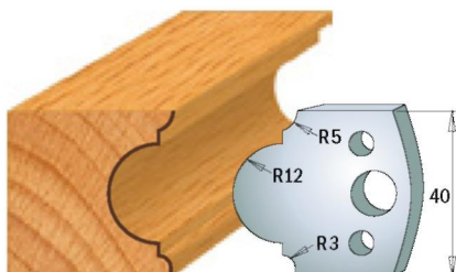
Пара ножів 690.018 Пара обмежувачів 691.018
