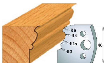
Пара ножів 690.101 Пара обмежувачів 691.101
