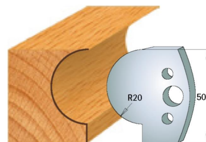
Пара ножів 690.562 Пара обмежувачів 691.562
