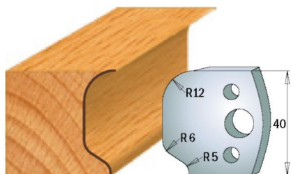
Пара ножів 690.048 Пара обмежувачів 691.048
