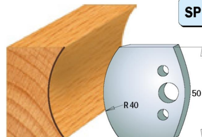
Пара ножів 690.553 Пара обмежувачів 691.553
