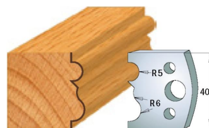
Пара ножів 690.029 Пара обмежувачів 691.029
