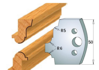
Пара ножів 690.542 Пара обмежувачів 691.542
