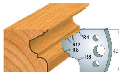
Пара ножів 690.089 Пара обмежувачів 691.089
