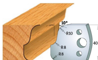
Пара ножів 690.059 Пара обмежувачів 691.059
