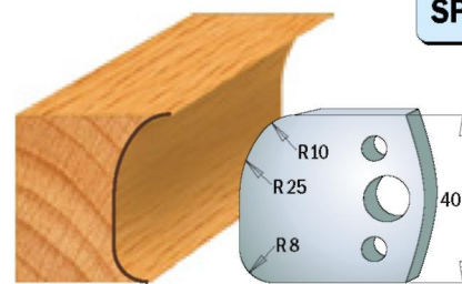
Пара ножів 690.062 Пара обмежувачів 691.062
