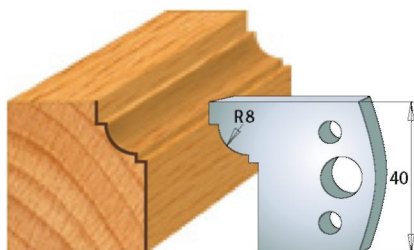
Пара ножів 690.067 Пара обмежувачів 691.067
