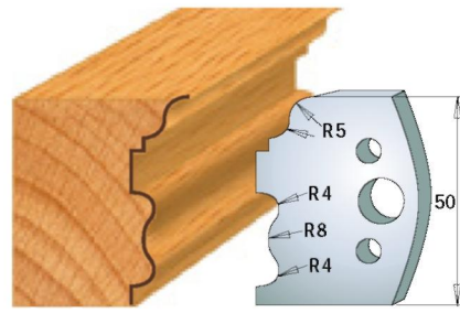
Пара ножів 690.515 Пара обмежувачів 691.515
