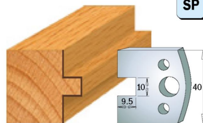
Пара ножів 690.092 Пара обмежувачів 691.092
