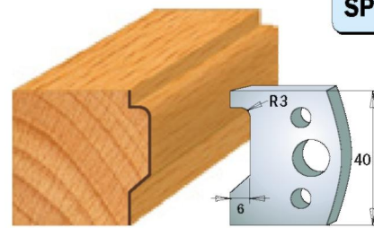
Пара ножів 690.032 Пара обмежувачів 691.032
