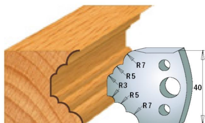
Пара ножів 690.021 Пара обмежувачів 691.021
