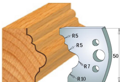
Пара ножів 690.508 Пара обмежувачів 691.508
