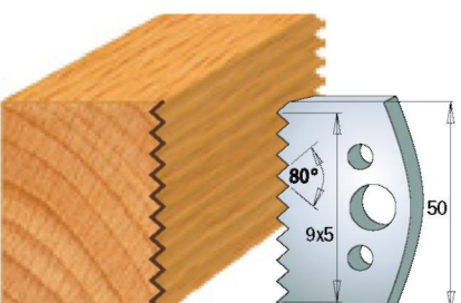
Пара ножів 690.524 Пара обмежувачів 691.524
