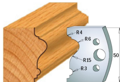
Пара ножів 690.512 Пара обмежувачів 691.512
