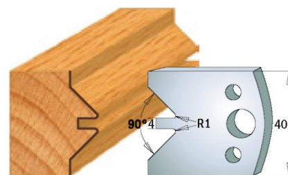
Пара ножів 690.071 Пара обмежувачів 691.071
