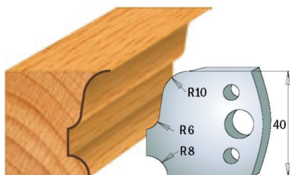
Пара ножів 690.064 Пара обмежувачів 691.064
