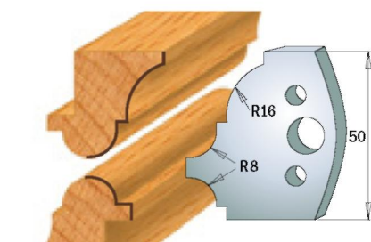
Пара ножів 690.541 Пара обмежувачів 691.541
