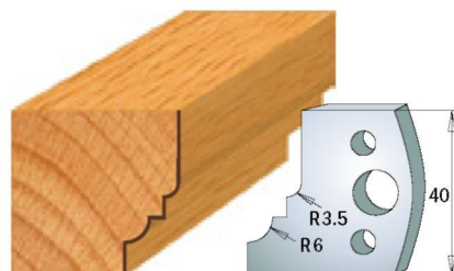
Пара ножів 690.019 Пара обмежувачів 691.019
