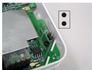
Датчик температуры помещения выключен (отсутствие якорька)
