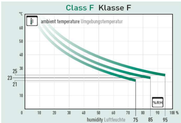
Limits of relative humidity of the ambient climate in relation to the ambient temperature. Grenzen der relativen Luftfeuchte des Kondensators in Abhängigkeit von der Umgebungstemperatur.
