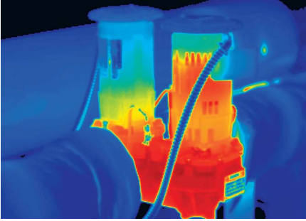
Рис. 5-66. Тепловые изображения можно использовать для определения работы каждой ступени двухступенчатого насоса.
