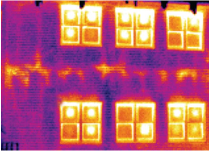
Рис. 5-50. Теплые участки в центре окон с двойным покрытием указывают на потерю теплоизолирующего аргона, который должен заполнять пространство внутри стеклопакетов.
