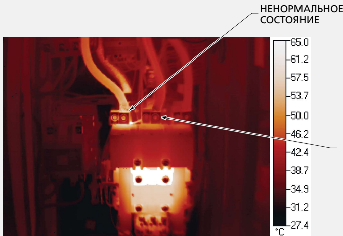
Рис. 2-1. Тепловые сигнатуры работающего оборудования могут быстро указать на нормальное и ненормальное состояние.
