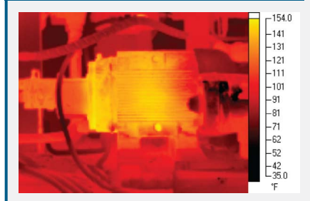
Рис. 7-2. Многие отличия тепловой сигнатуры двигателя проявятся при последующих обследованиях.
