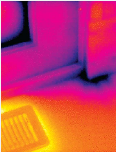
Рис. 6-6. Тепловые следы, связанные с течами воздуха, часто имеют характерный «размытый» вид.
