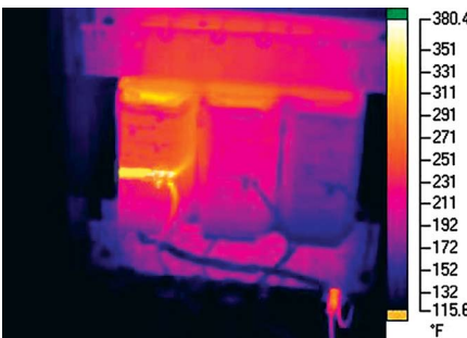
Рис. 5-58. Тепловое изображение трехфазного сухого трансформатора показывает, что основной вывод на левой фазе имеет ненормальный нагрев.
