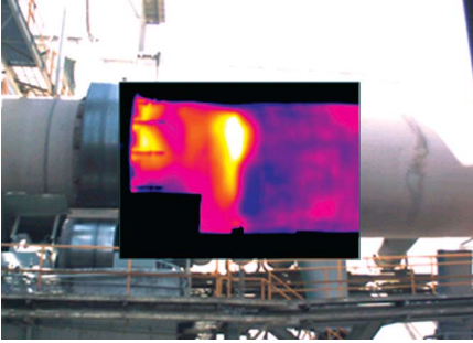
Рис. 5-9. Тепловидение можно использовать для контроля состояния футеровки во времени и выявлять проблемные зоны в цементных печах и другом промышленном оборудовании.
