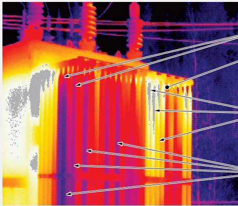
Рис. 4-2. Естественная конвекция наблюдается, когда теплое масло поднимается вверх, а холодное опускается вниз, как происходит в охлаждающих трубках маслонаполненного трансформатора.
