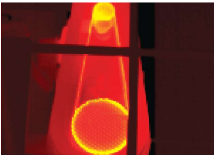
Рис. 5-74. Светлые области на тепловом изображении ремня и шкивов указывают на возможные проблемы соосности.
