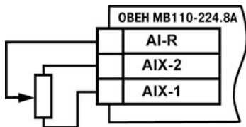
Рисунок 3.4 – Схема подключения резистивного датчика к входу прибора
