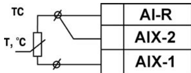
Рисунок Б.2 – Схема подключения термометра сопротивления
