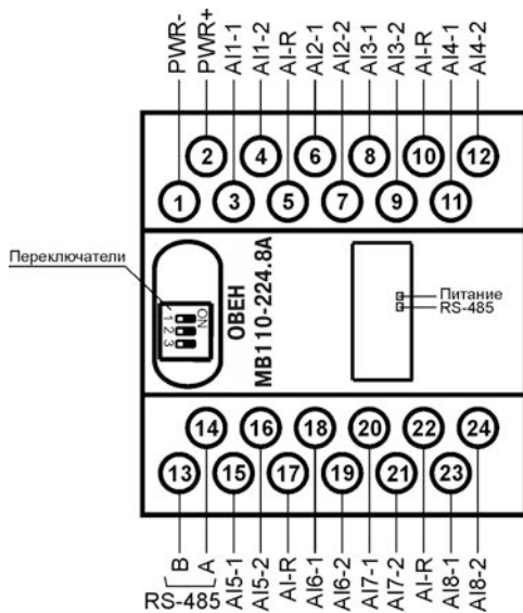
Рисунок Б.1 – Общий чертеж прибора
