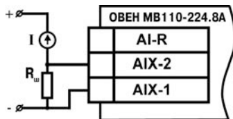
Рисунок 3.3 – схемы подключения активного датчика с токовым выходом к входу прибора
