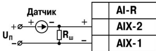
Рисунок Б.5 – Схема подключения активного датчика с токовым выходом 0...5,0, 0...20,0 или 4...20,0 мА ( R_{ш}=50,000 \pm 0,025 Ом)
