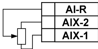
Рисунок Б.6 – Схема подключения датчика положения резистивного типа 0...900 Ом или 0...2000 Ом
