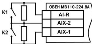
Рисунок 3.5 – Схема подключения «сухих контактов»
