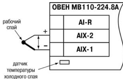
Рисунок 3.2 – Схема подключения ТП к входу прибора
