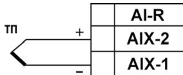
Рисунок Б.3 – Схема подключения термоэлектрического преобразователя
