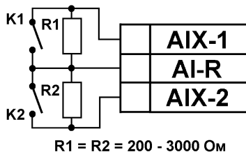
Рисунок Б.7 – Схема подключения дискретных датчиков «сухие контакты»
