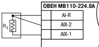
Рисунок 3.1 – Схема подключения ТС к входу прибора
