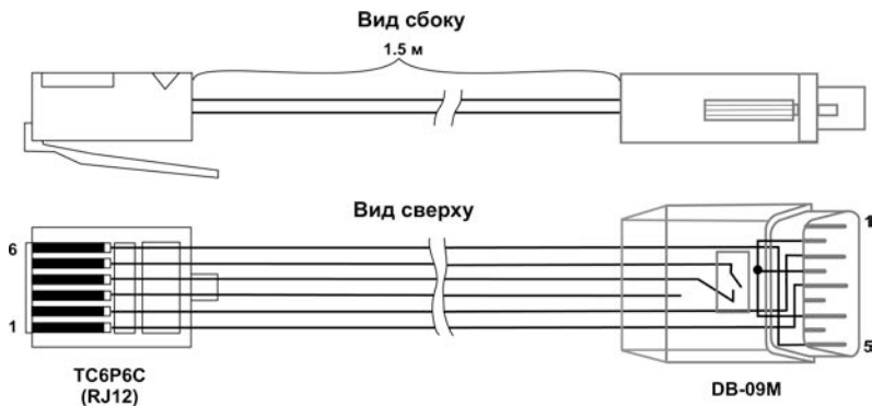
Рисунок Б.5 – Схема "Модемный кабель ПЛК1ХХ"
