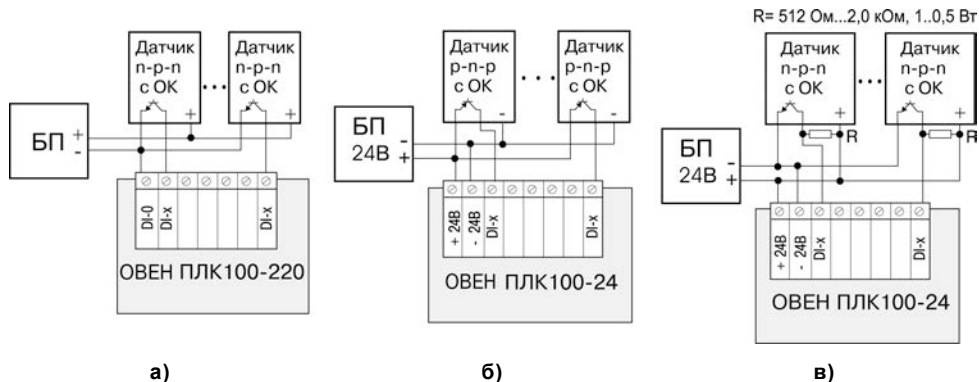
Рисунок Б.8 – Схемы подключения к ОВЕН ПЛК100 дискретных датчиков с полупроводниковым выходным каскадом: а) ОВЕН ПЛК100-220 датчик n-p-n-типа, б) ОВЕН ПЛК100-24 датчик p-n-p-типа, в) ОВЕН ПЛК100-24 датчик n-p-n-типа
