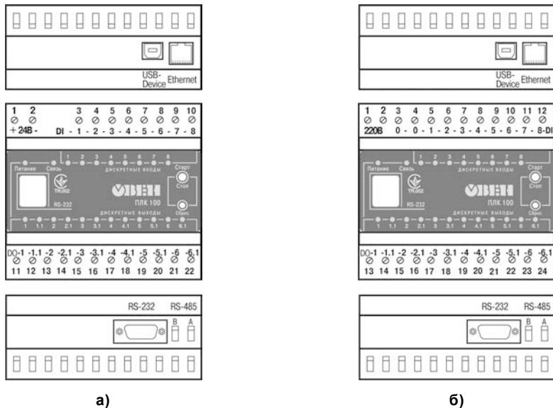
Рисунок 3.1 – Внешний вид ОВЕН ПЛК100-24 (а) и ОВЕН ПЛК100-220 (б)
