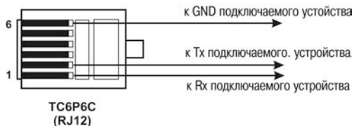
Рисунок Б.7 – Схема кабеля для подключения к порту Debug RS-232
