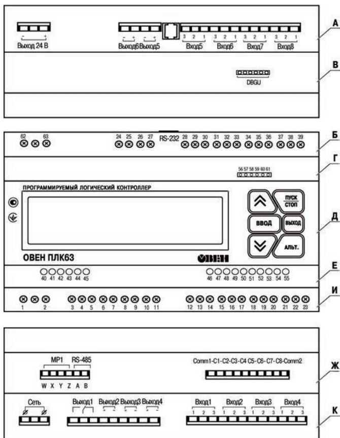
Рисунок 3.1 – Разъемные соединения, элементы индикации и управления контроллера
