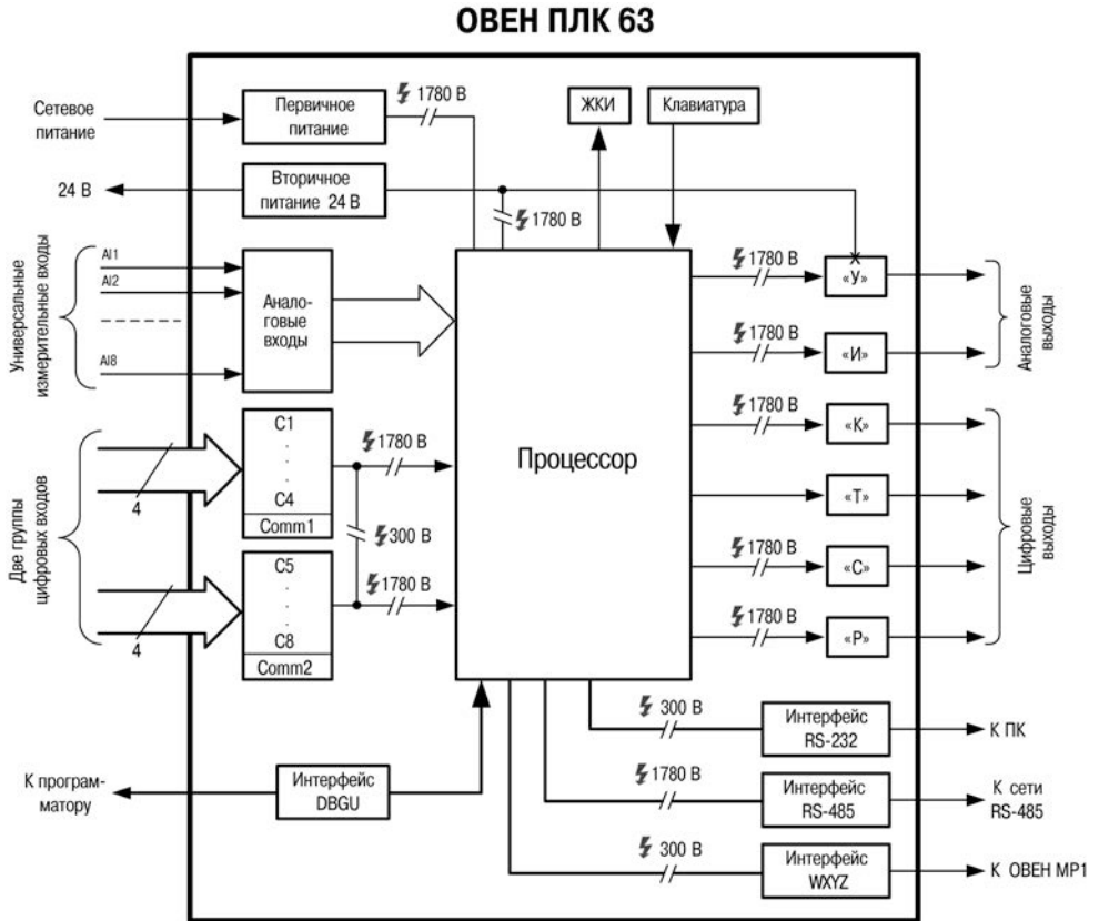
Рисунок 3.2 – Функциональная схема контроллера
