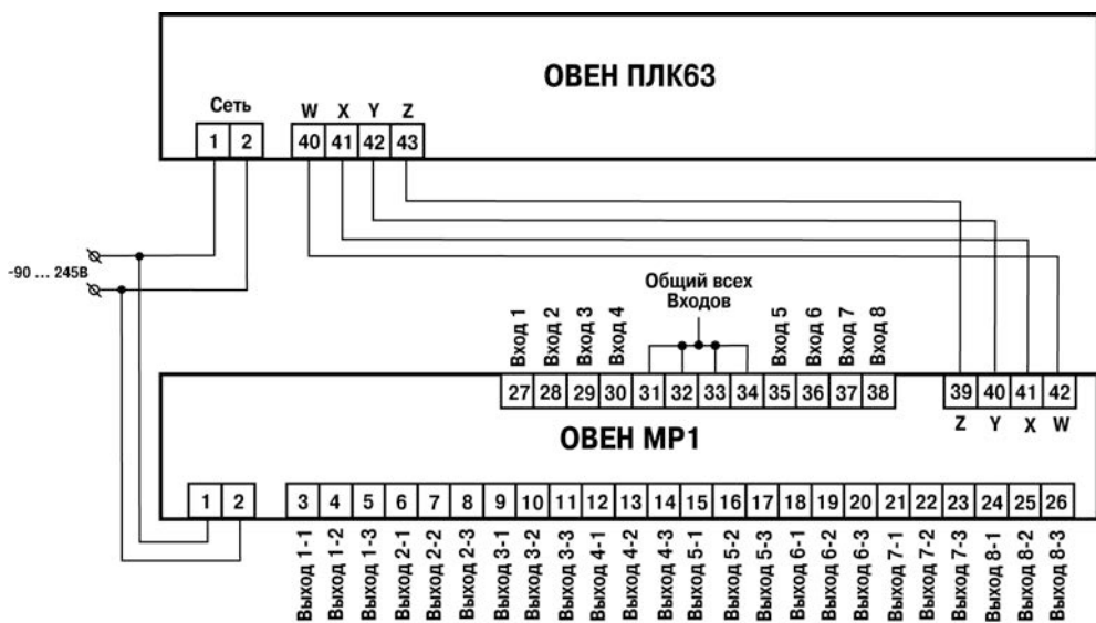
Рисунок Б.15 – Схема подключения модуля ОВЕН МР1 к контроллеру
