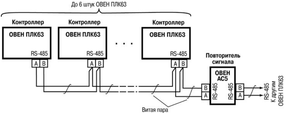
Рисунок 6.3 – Пример схемы подключений в сеть более 6-ти ОВЕН ПЛК63 (ОВЕН АС5 – повторитель сигнала)
