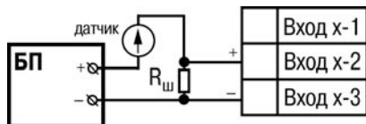
Рисунок Б.5 – Подключение активного датчика с токовым выходом 0...5 \text{ мА} или 0(4)...20 \text{ мА} ( R_{ш} = 100,0 \text{ Ом} \pm 0,1\% )
