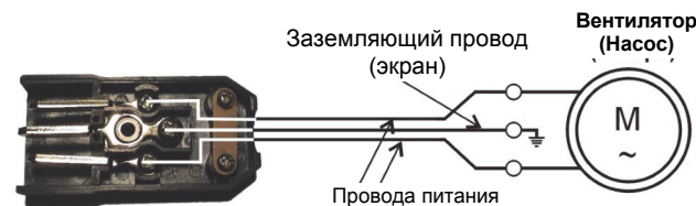
Рис. Подсоединение проводов от вентилятора/насоса к вилке
