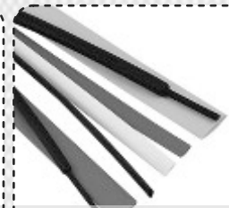
Трубка термоусаживаемая с коэффициентом усадки 2:1, подавляющая горение (НГ)
