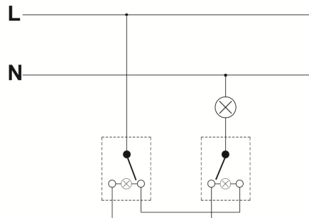
Łącznik schodowy z podświetleniem
