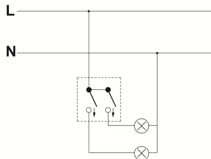
Łącznik świecznikowy
