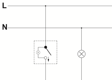
Łącznik jednobiegunowy z podświetleniem
