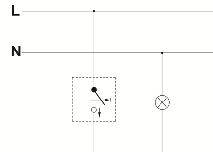
Łącznik zwierny (dzwonek, światło)
