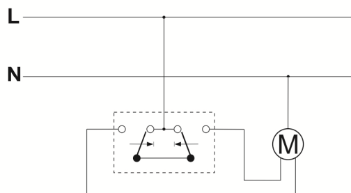
Łącznik żaluzjowy
