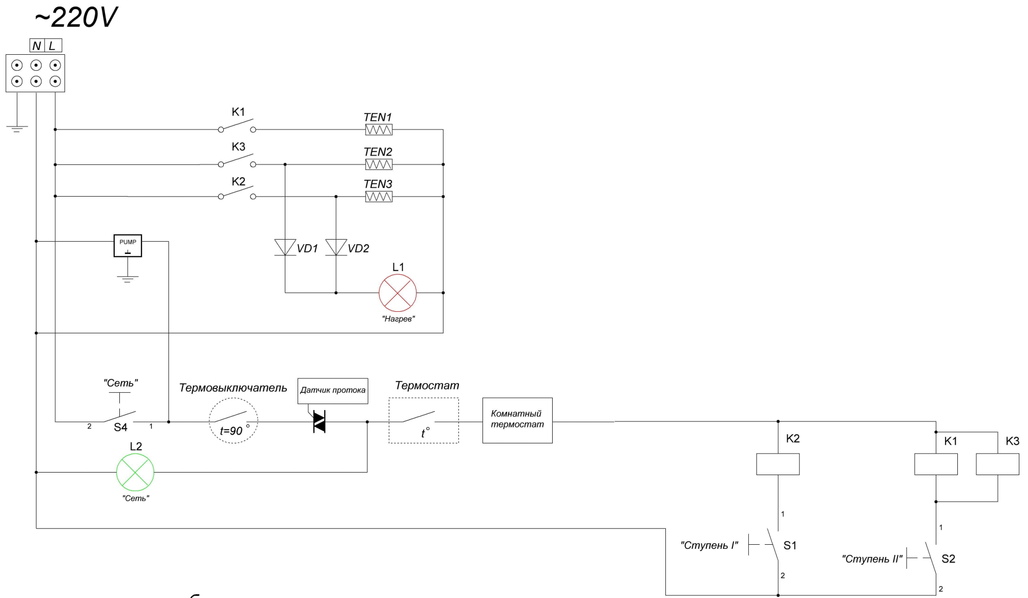
Схема электрическая принципиальная котла "Стандарт"
