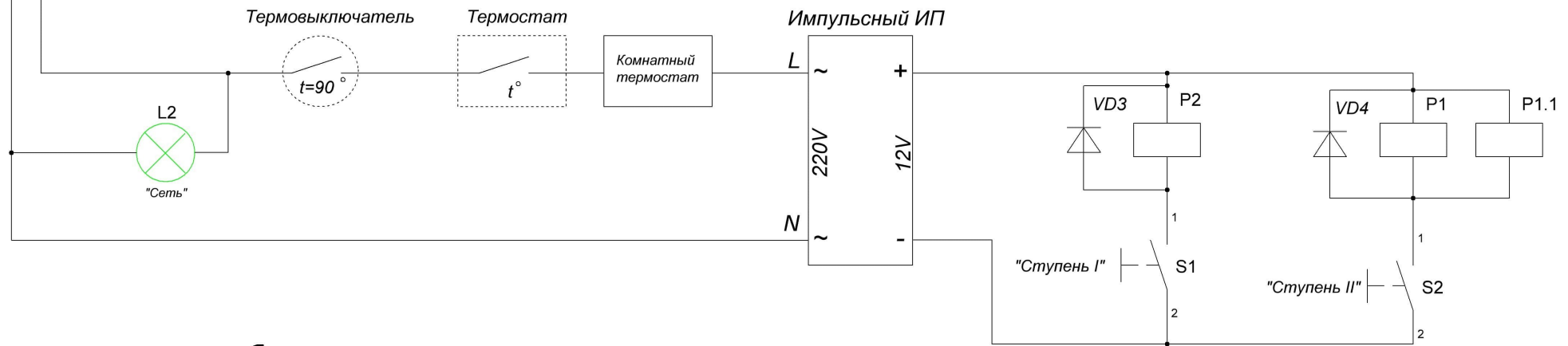
Схема электрическая принципиальная котла "Эконом"
