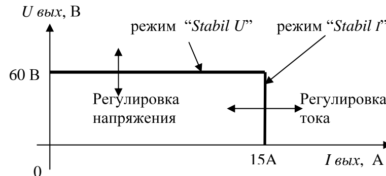
Рис. 4. Вольтамперная характеристика источника питания
