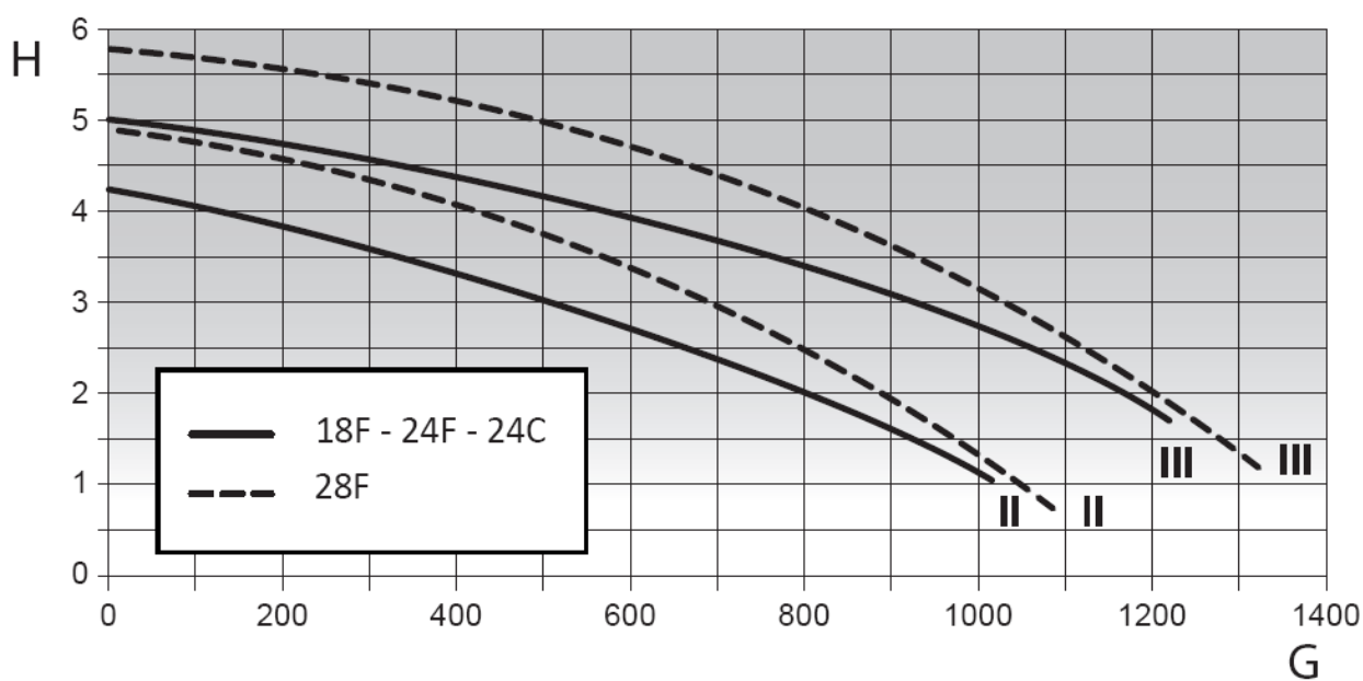
Насос котла Oberon
