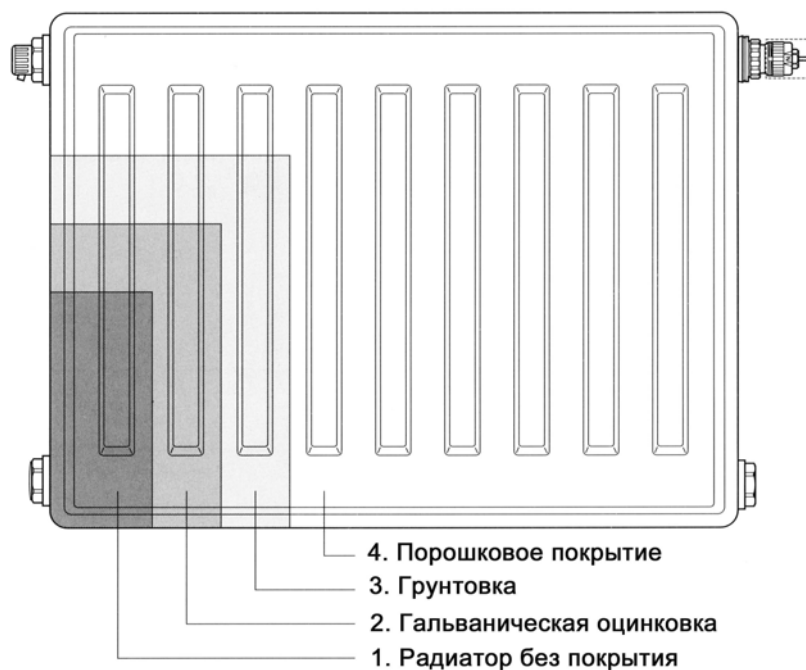
Рис. 1.3. Последовательность покрытия оцинкованных радиаторов «VONOVA»
