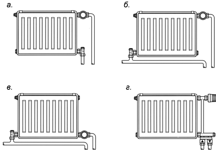
Рис. 2.2. Варианты присоединения радиаторов «VONOVA Компакт» с термостатами фирмы «ГЕРЦ» при напольной или плинтусной разводке теплопроводов
