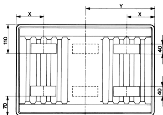
Рис. 6.1. Схема расположения скоб для крепления радиаторов всех типов на стене
