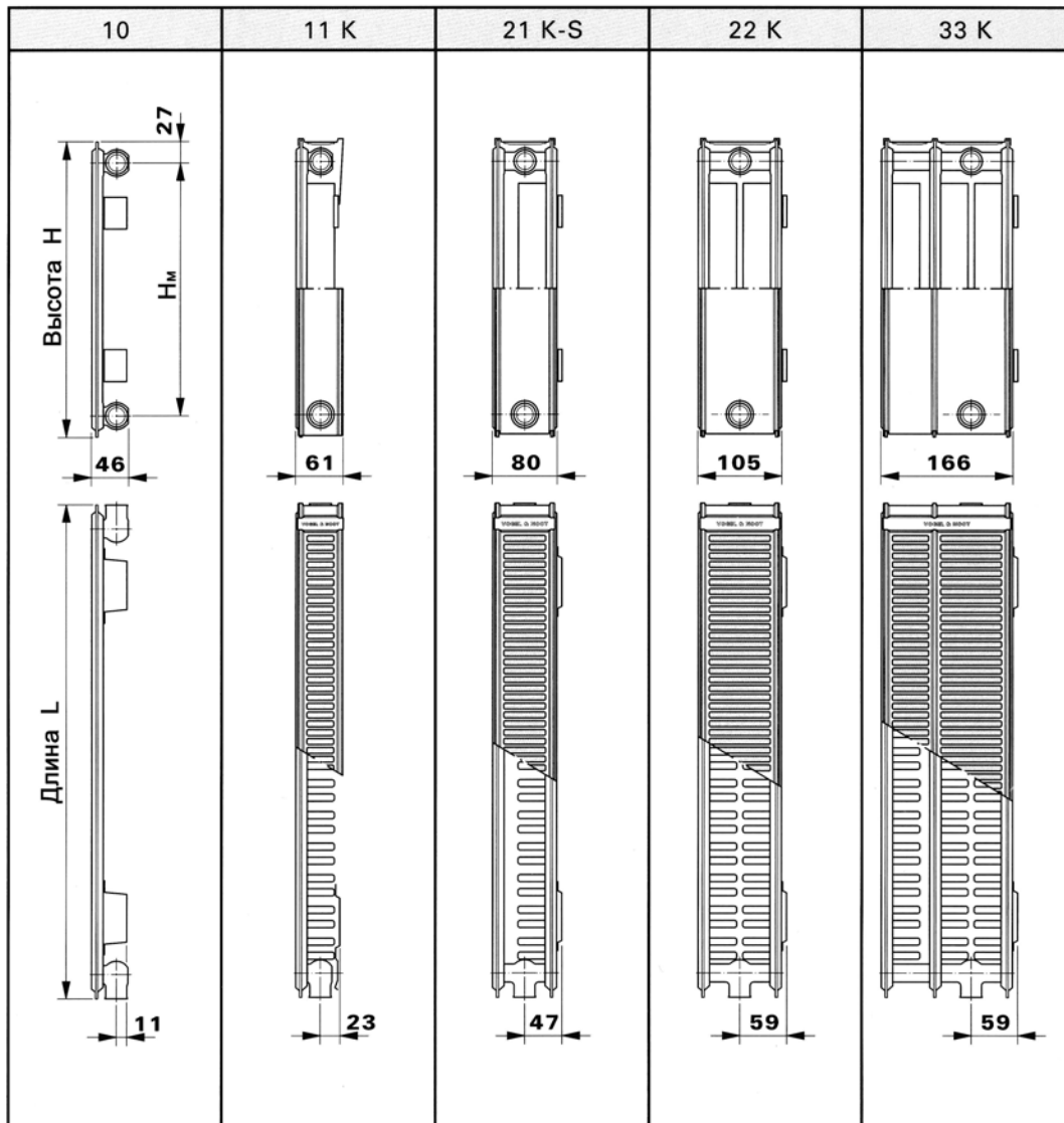
Рис. 1.2. Номенклатура радиаторов «VONOVA Kompakt»
