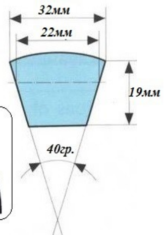
Ремень профиль D(Г)
