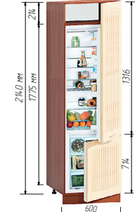
Шкаф для двухкамерного встроенного холодильника
