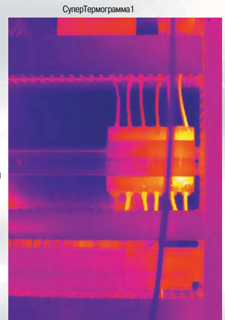
СуперТермограмма 1 Разрешение 320 x 240 пикселей
