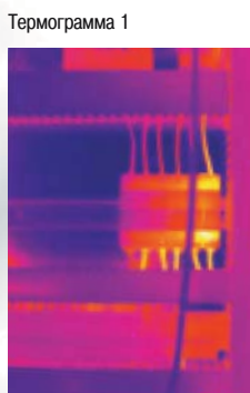
Термограмма 1 Разрешение 160 x 120 пикселей
