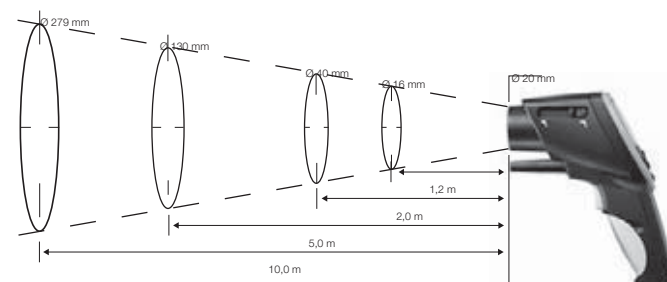
Диаметр измерительной точки при различных расстояниях от измеряемой поверхности
