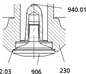
412.03 906 230 Рисунок 23: Демонтаж рабочего колеса
