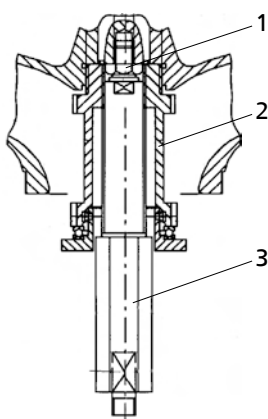
Рисунок 26: Съёмник
