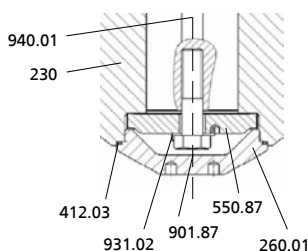
940.01 230 412.03 931.02 901.87 550.87 260.01 Рисунок 24: Демонтаж рабочего колеса
