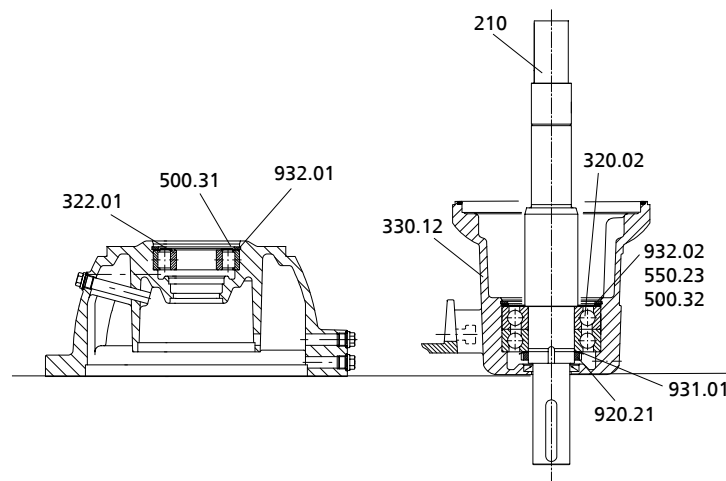
Рисунок 31: Демонтируйте вал
