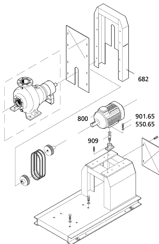
Рисунок 21: Демонтаж ремня
