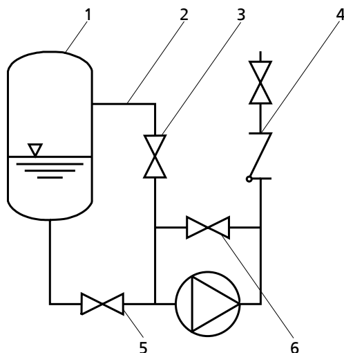
Рисунок 7: Компенсация вакуума
